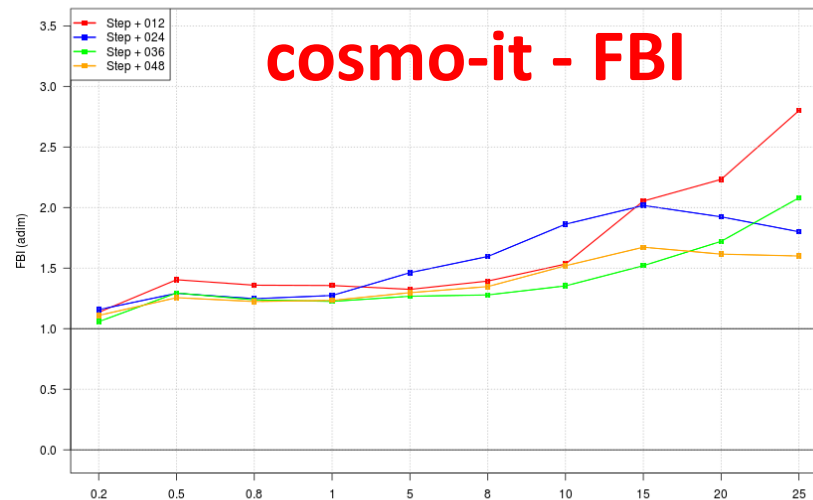
COSMO-IT - Prec06h - SON 2024 - All ITA stations
