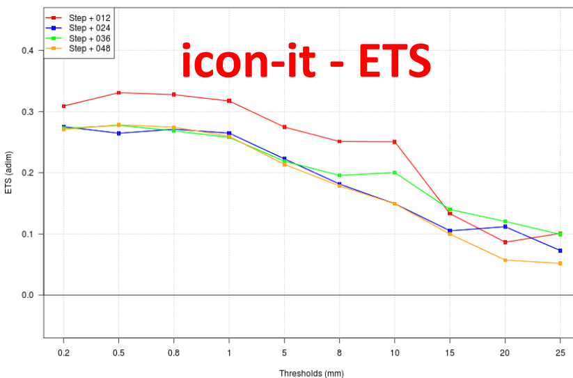
ICON-IT - Prec06h - SON 2024 - All ITA stations
