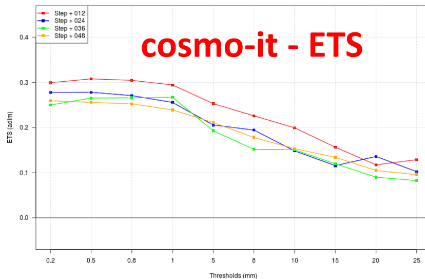
COSMO-IT - Prec06h - SON 2024 - All ITA stations
