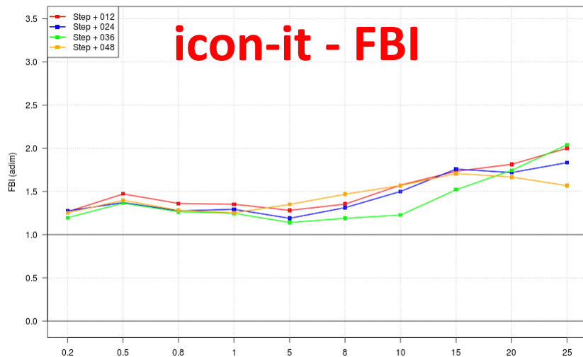
ICON-IT - Prec06h - SON 2024 - All ITA stations
