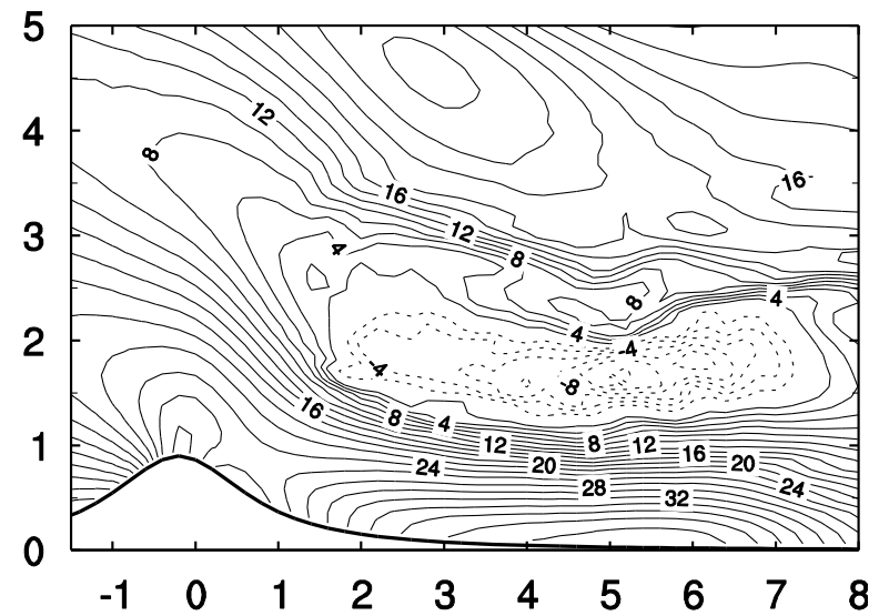
CE-C-Explicit
