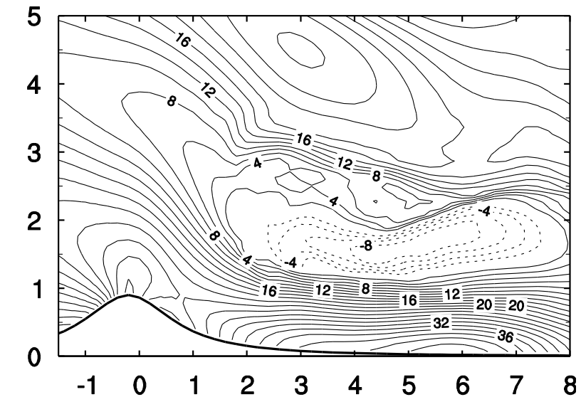
CE-A
